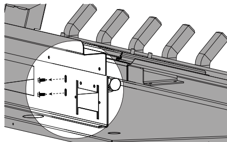
FIG. 2: Vue de Côté/Arrière de l'Assemblage du Brûleur
